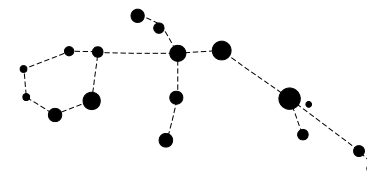
Constelación de Acuario
