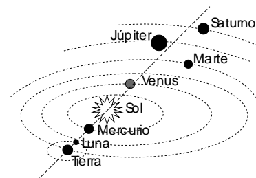
Alineación de los Planetas el 4 de Febrero del 1962
