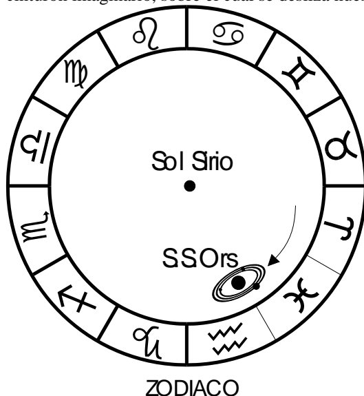
Alineación de los Planetas el 4 de Febrero del 1962
